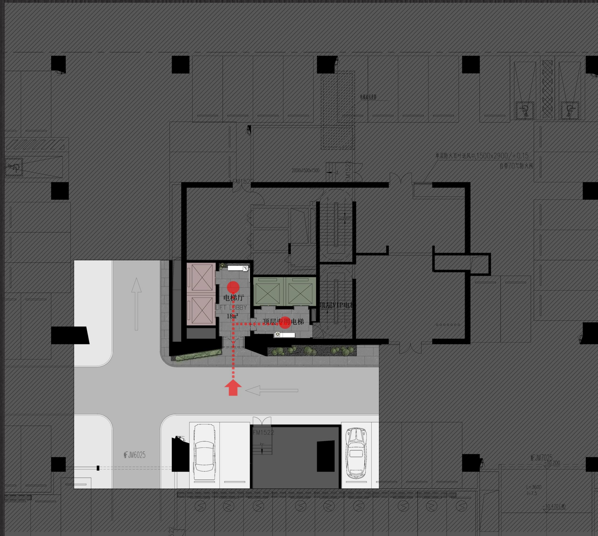
B2平面图
